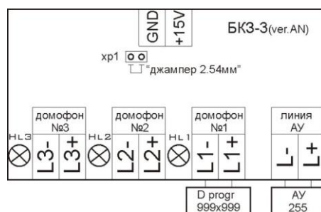
Рис.2 «Программирование»
